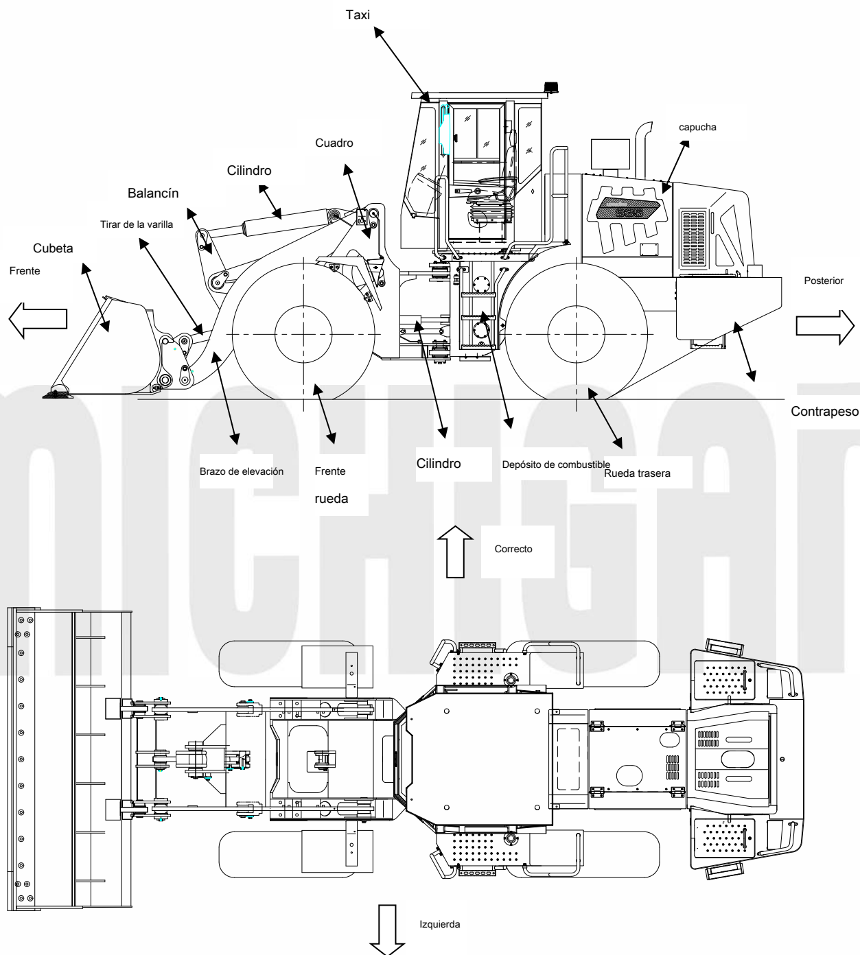
Diagrama esquemático de componentes del cargador
