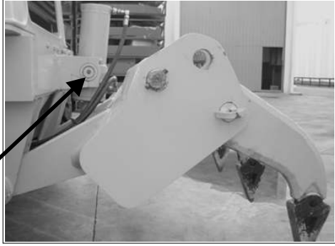
Cilindro escarificador
